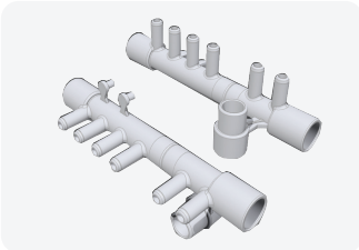
Part #: 72016 (6) 3/8"SB x (2) 1/2"S
